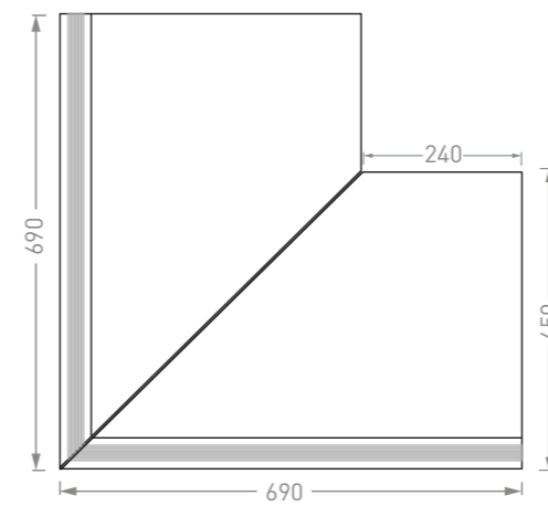
MIKONOS EDGE 45X70 CM BORDE MIKONOS 45X70 CM Ref. BPMI EE00 E2C 45X70 [2 uds.]
