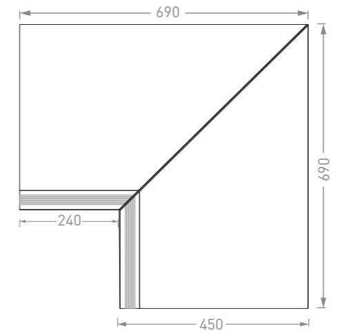
MIKONOS EDGE 45X70 CM BORDE MIKONOS 45X70 CM Ref. BPMI EI00 E2C 45X70 [2 uds.]
