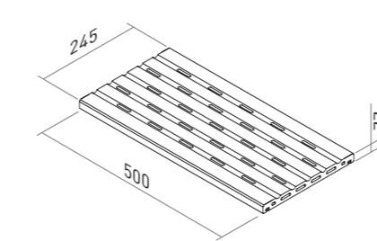
CERAMIC DRAIN GRATE REJILLA DE DRENAJE CERÁMICA Ref. RJ67 0000 25x50 (M-780) pz MONOBLOCK
